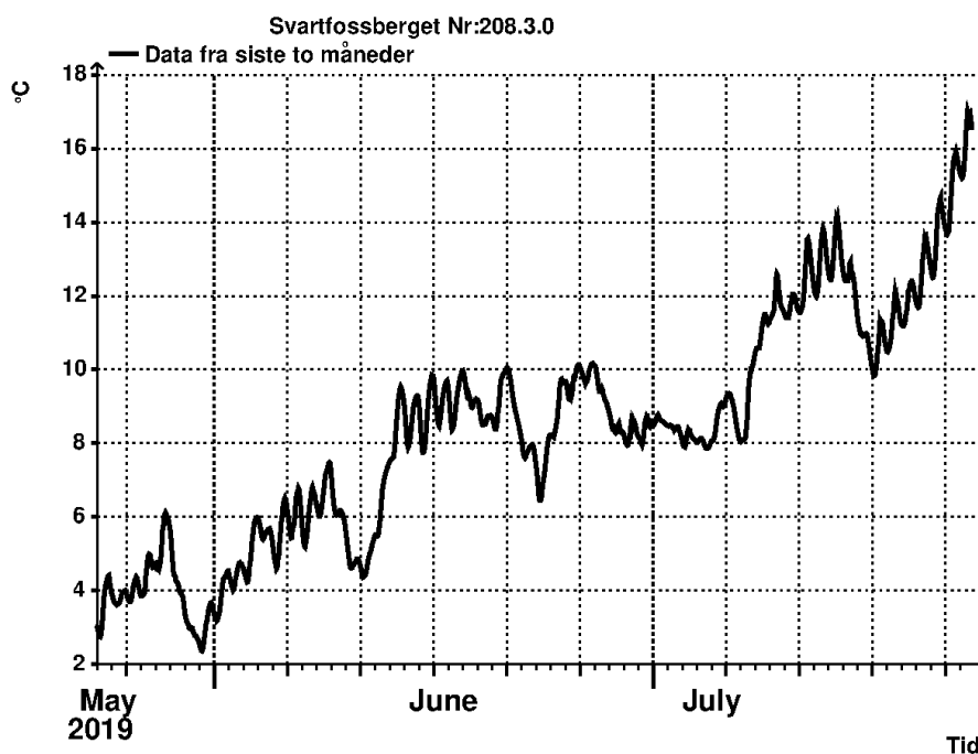
Figur 3: Vanntemperaturen i Reisaelva sesongen 2019.
