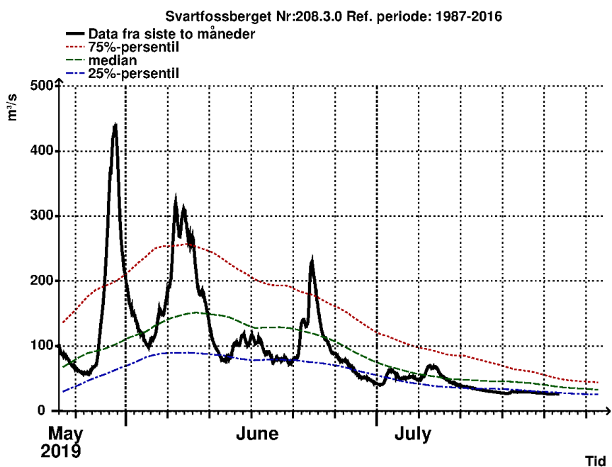
Figur 2: Vannføringen i Reisaelva sesongen 2019.
