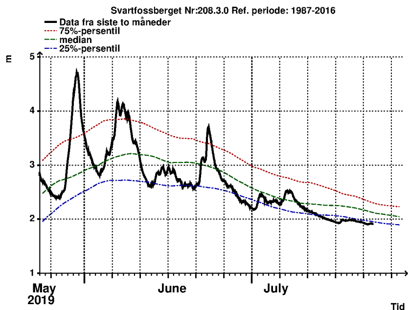
Figur 1: Vannstanden i Reisaelva ved målestasjonen ved Svartfossberget fra mai 2019 frem til 22. juli.
